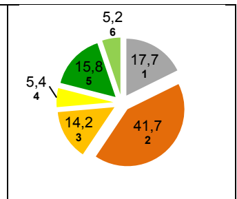
Energieträgermix Deutschland
