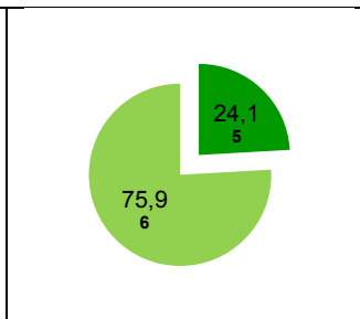
Energieträgermix Ökostrom-Produkt **
