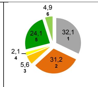
Energieträgermix Normalstrom-Produkte *
